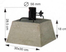
RESORT STAND Size S/NW. 30 Kgs. (แบบกลางรุ่นสี)
