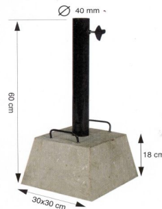
RESORT STAND Size S/NW. 30 Kgs. (แบบกลางรุ่นขาว)
