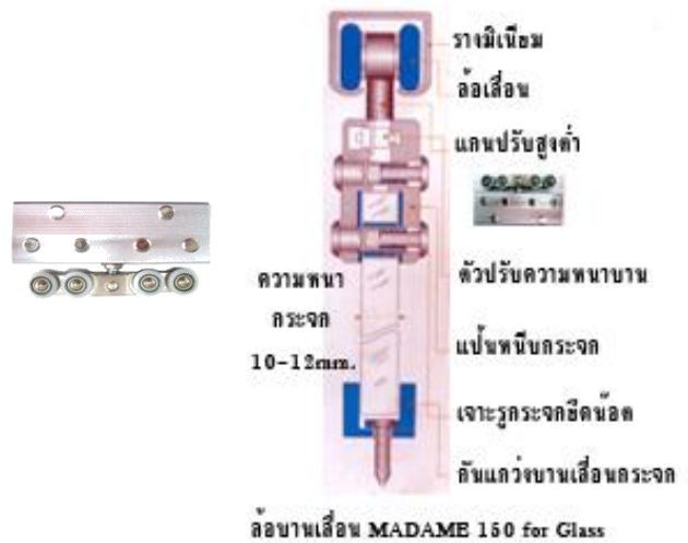
ล้อบานเลื่อนกระจก MADAME/150 รับน้ำหนัก 150 kg. ต่อบาน
