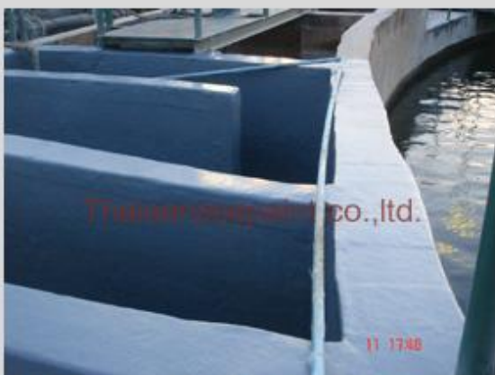
ชื่องาน :งานเคลือบ FRP พื้นที่ใช้งาน :บ่อบำบัดน้ำเสีย Location :นิคมฯ มาบตาพุด
