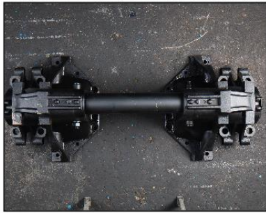
15..... แท่นเพลลาโบกี้ ISUZU .....
